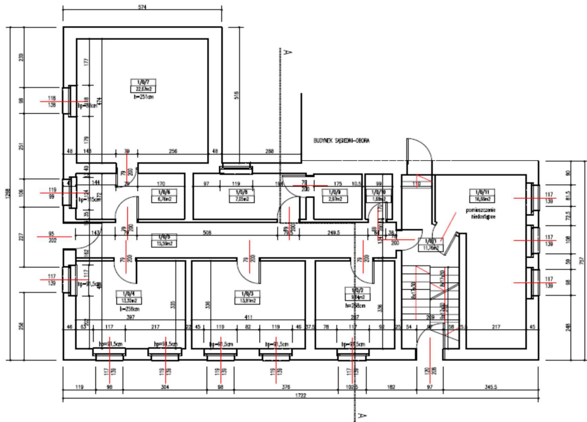
RZUT PARTERU
